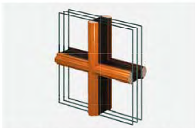
Aufgeklebte Zierfalzsprosse (24 mm) aussen und Zierfalz- sprosse innen mit zwei innenliegenden Abstandhaltern
