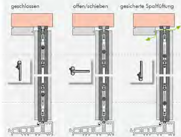
Bedienung und Funktionalität – bekannte Griffstellungen und Spaltlüftung
